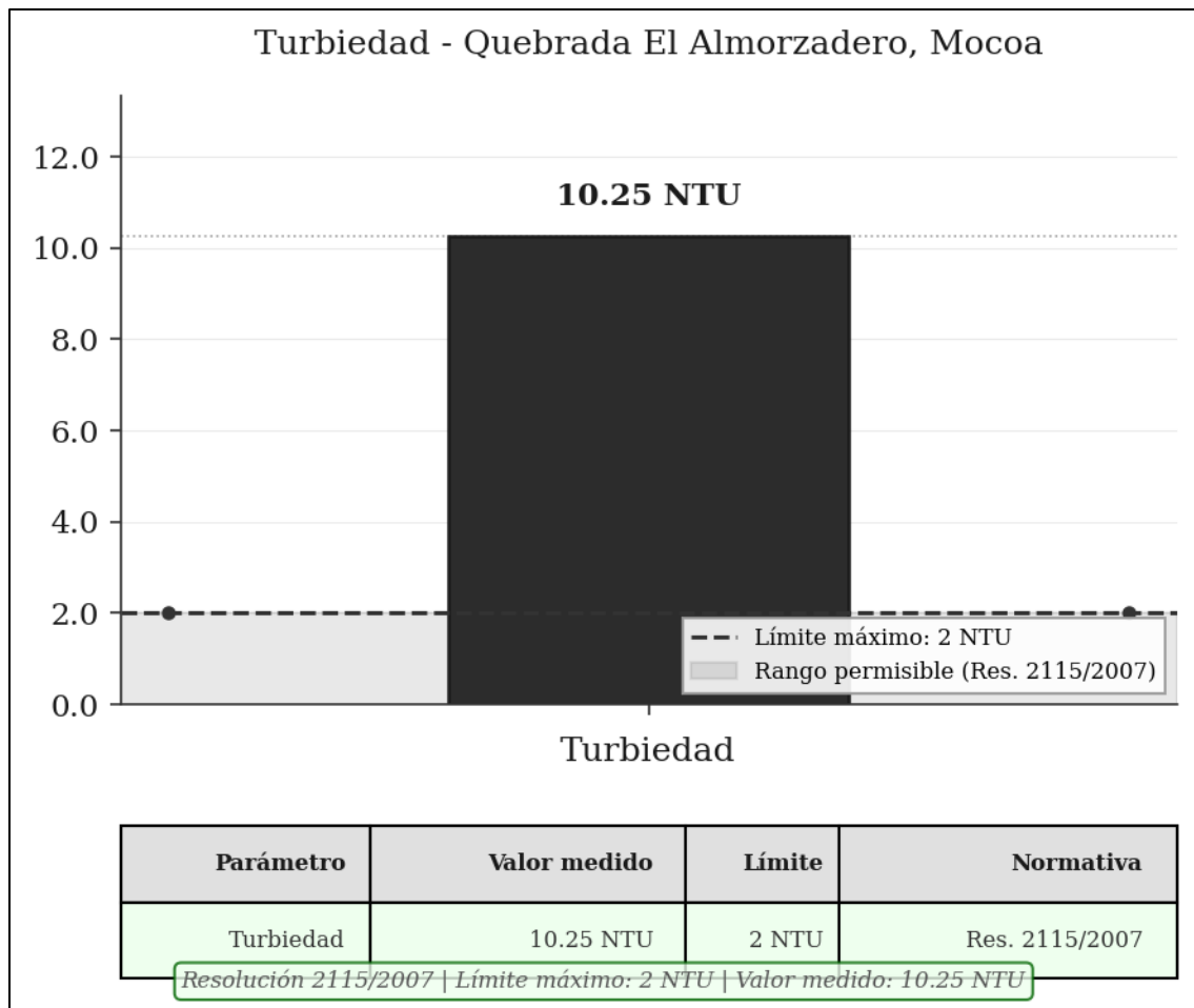
Figura 12 Grafico valores Turbiedad
