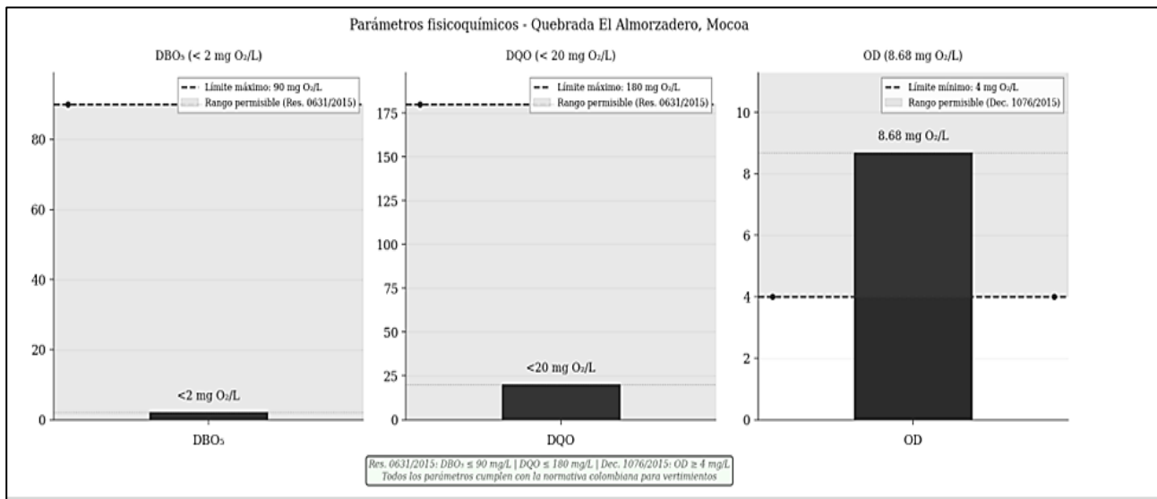
Figura 8 Grafico valores DBO 5 , DQO y OD
